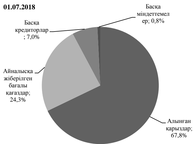
2-график. Ипотекалық ұйымдар міндеттемелерінің құрылымы
